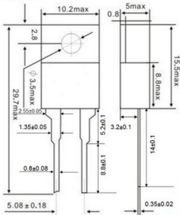
JUC-31F温控器开关规格图纸
