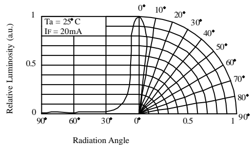
Directivity (Angle : 15°)
