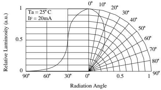
Directivity (Angle : 60°)
