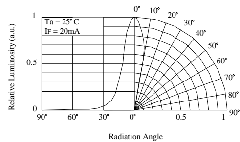
Directivity (Angle : 20°)
