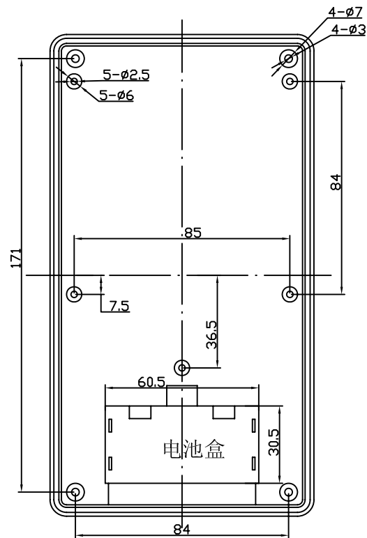
下盖正视图
