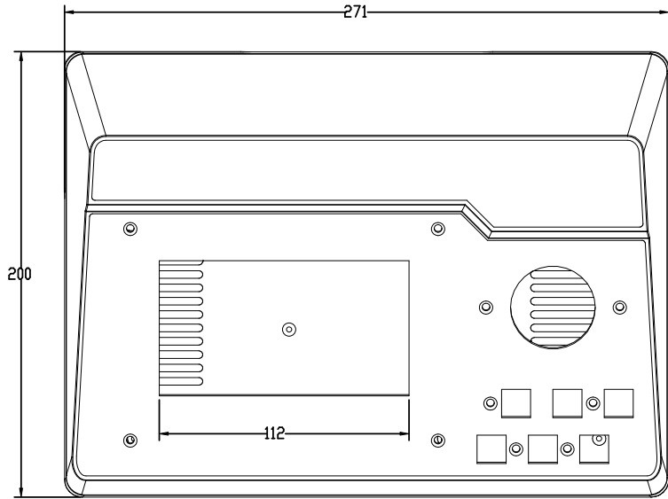
下盖正视图
