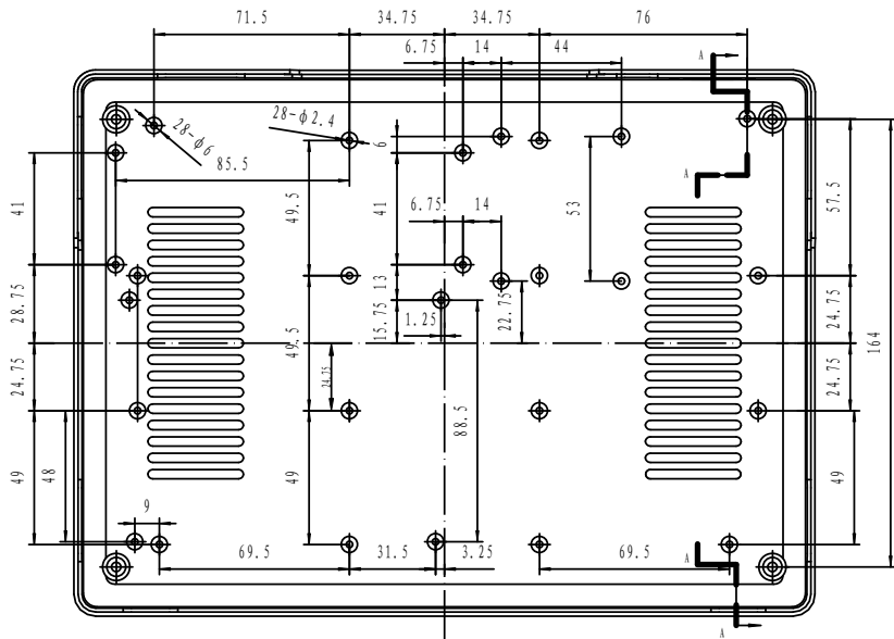
下盖正视图
