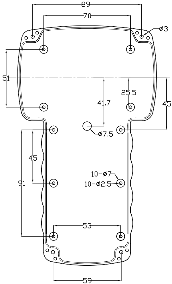
下盖正视图
