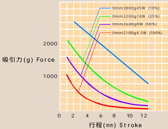
行程/吸引力 Stroke and Force
