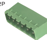
X977201 5mm Female terminal block (right angle) A: 2P B: 3P C: 4P D:5P E: 6P F: 7P G: 8P H:9P J:10P K:11P L:12P
