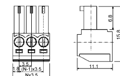
X977221 3.5mm Female terminal block (right angle) A: 2P B: 3P C: 4P D:5P E: 6P F: 7P G: 8P H:9P J:10P K:11P L:12P
