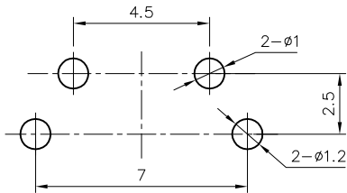
PCB. 焊接图
