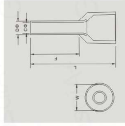
尼龙绝缘护套管形端子(适用于软线)
