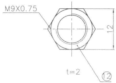
Nut 1PC
